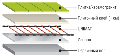
Рис. 25. Схема монтажа теплого пола UNIMAT под плитку/керамогранит
