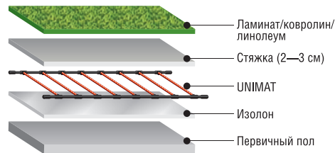
Рис. 23. Схема монтажа теплого пола UNIMAT под ламинат/ковролин/ линолеум
