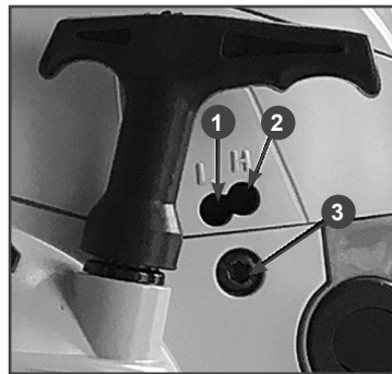
Рис. 20 Винты регулировки карбюратора
